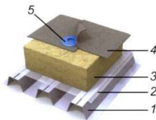
1. att. Savietotā lēzenā juma konstrukcija ar vienslāņa siltumizolāciju: 1 – nesošā profilētā tērauda loksne; 2 – tvaikizolācija (speciālā polietilēna plēve); 3 – cietās akmens vates plāksne ROS 40; 4 – ruļļmateriālu jumta segums; 5 – mehāniskais stiprinājuma elements
