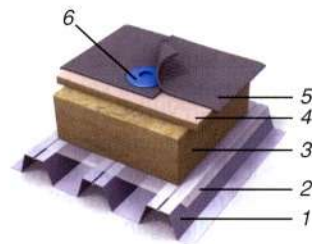
2. att. Savietotā lēzenā juma konstrukcija ar divslāņu siltumizolāciju: 1 – nesošā profilētā tērauda loksne; 2 – tvaikizolācija (speciālā polietilēna plēve); 3 – cietās akmens vates plāksne ROS 30; 4 – īpaši cietās akmens vates plāksne ROB 50; 5 – ruļļmateriālu jumta segums; 6 – mehāniskais stiprinājuma elements
