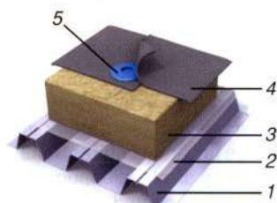
1. att. Savietotā lēzenā juma konstrukcija ar vienslāņa siltumizolāciju: 1 – nesošā profilētā tērauda loksne; 2 – tvaikizolācija (speciālā polietilēna plēve); 3 – cietās akmens vates plāksne ROS 40; 4 – ruļļmateriālu jumta segums; 5 – mehāniskais stiprinājuma elements
