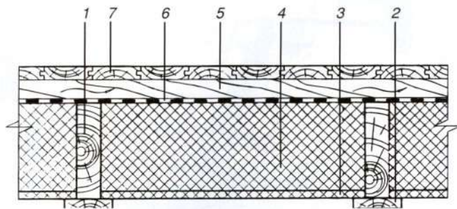
1. att. Koka vai parketa dēļu grīdas konstrukcija ar auksto pagrīdi: 1 – sija; 2 – koka dēlis; 3 – pretvēja plāksne; 4 – mikstās akmens vates plāksnes; 5 – gulšnis; 6 – tvaikizolācija; 7 – koka vai parketa dēļu grīda
